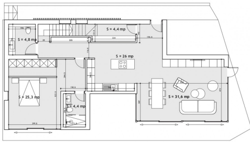
PLANTA BAJA
